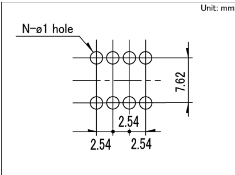
安装孔尺寸图
